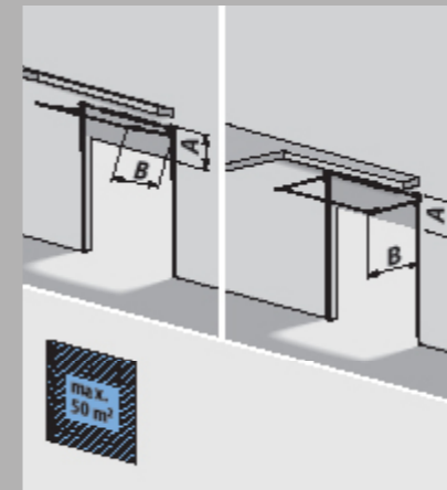
T 400 (B350), förhöjt skensystem
