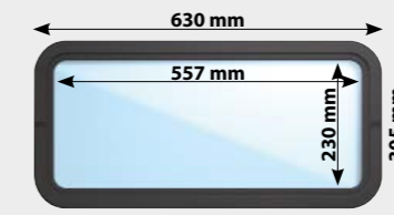
Rundade hörn (r=60 mm), utmärkt isolerande värde
