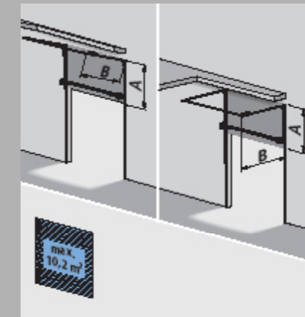
T 400 DS (B350 lastbrygga), höglyftande skensystem med nedflyttad fjäderaxel
