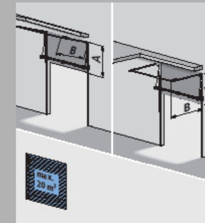
T 400 hF (B350), höglyftande skensystem med nedflyttad fjäderaxel + ståltub
