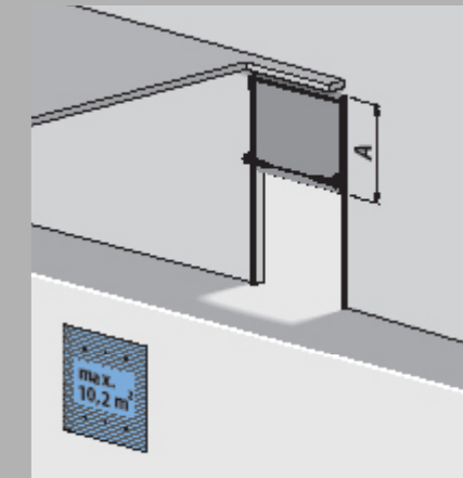
T 500 DS (B550 dock), nedflyttad fjäderaxel + ståltub med nedflyttad fjäderaxel
